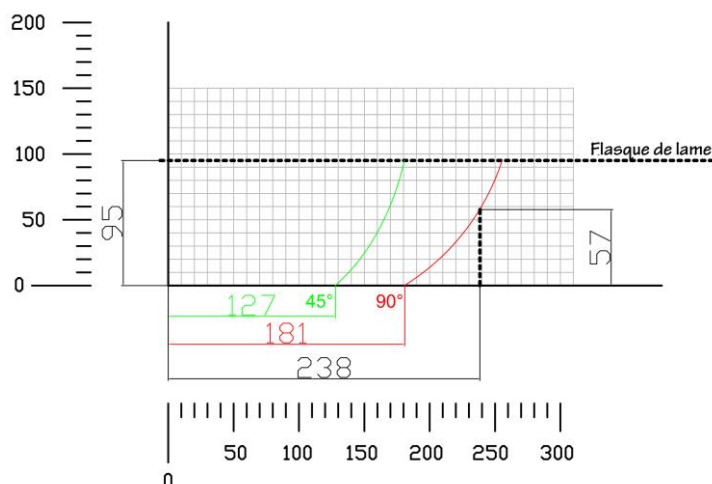
Diagramme de coupe (tolérance +/- 3 mm)
