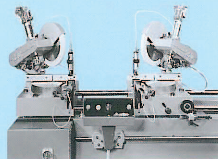
Lames en position pour une coupe à 45°
