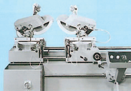
Position des lames lors d'une coupe biaisée débillardée
