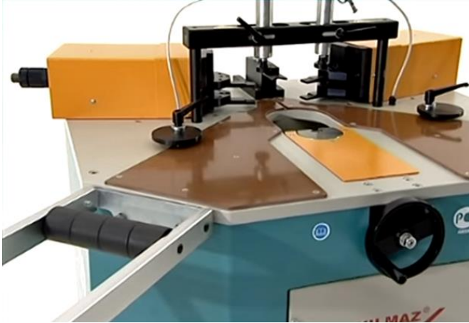
Détails des butées et des poinçons
