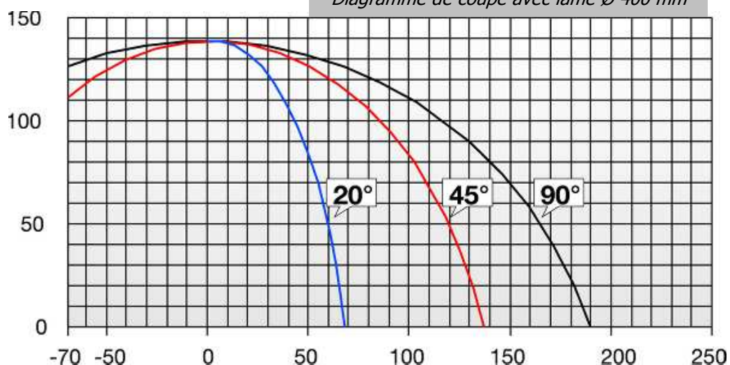
Diagramme de coupe avec lame Ø 400 mm
