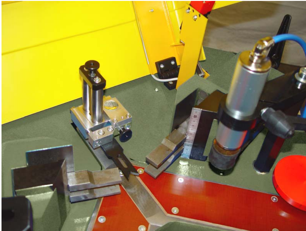
Détails des butées et du poinçon
